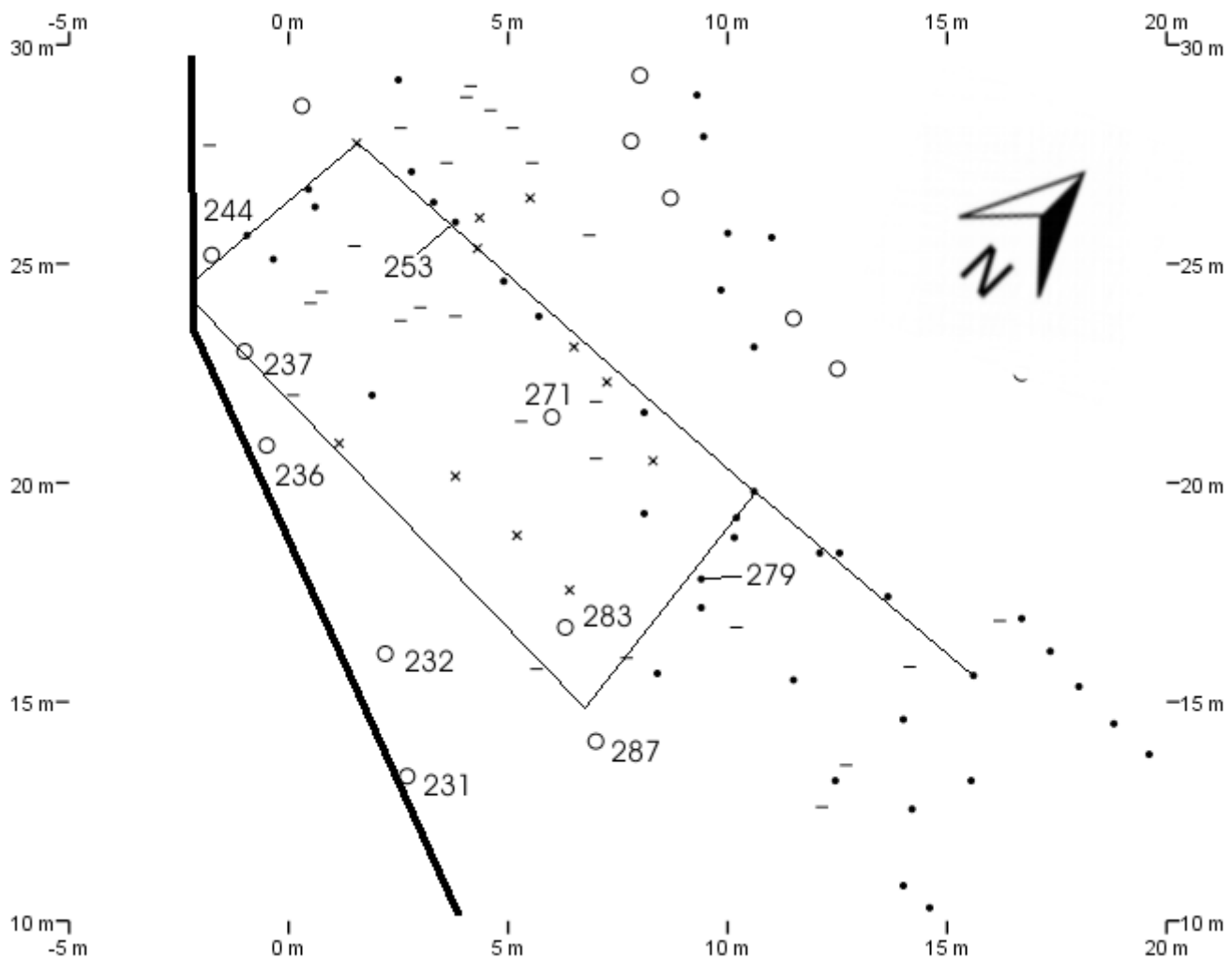
Abb. 145: Hüllhorst 2001/2002, Haus 7.
