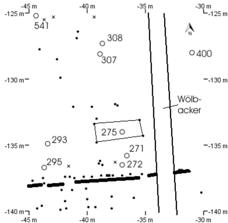
Abb. 159: Kirchlengern, Speicher 3.
